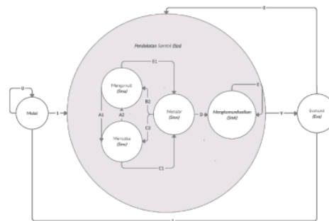
Gambar 12. Gameplay SG tematik SD dalam bentuk HFSM.
