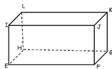
Gambar 2. Bangun Ruang Balok
