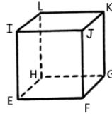
Gambar 1. Bangun Ruang Kubus
