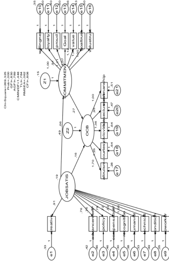
Gambar 4.1 Model SEM
