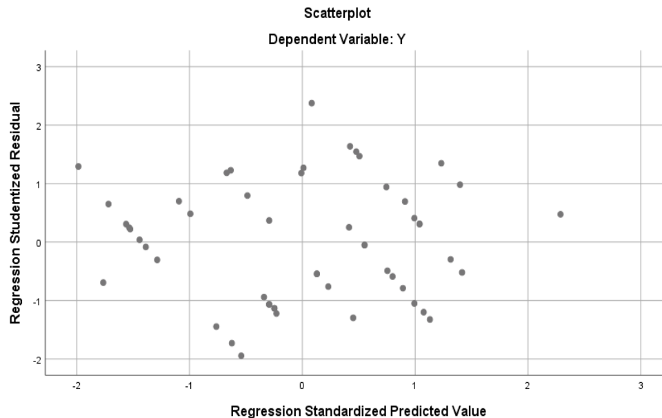
Gambar 4.1 Uji Heteroskedastisitas
