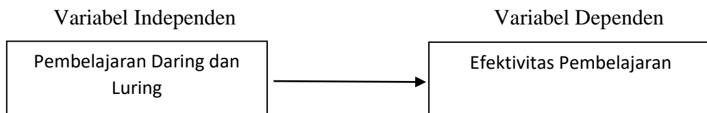
GAMBAR III. 2 Kerangka Konsep
