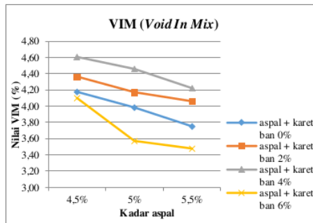
Gambar 11. Grafik nilai VIM
