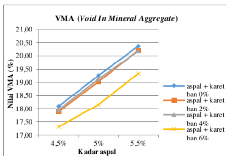
Gambar 12. Grafik nilai VMA
