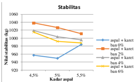
Gambar 15. Grafik nilai stabilitas
