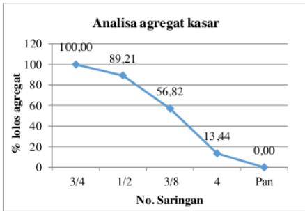
Gambar 9. Hasil analisa saringan agregat kasar
