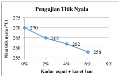
Gambar 5. Hasil pengujian titik nyala
