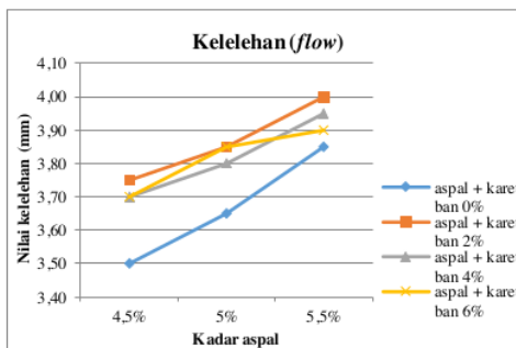
Gambar 14. Grafik nilai flow
