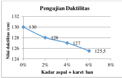
Gambar 4. Hasil pengujian daktilitas
