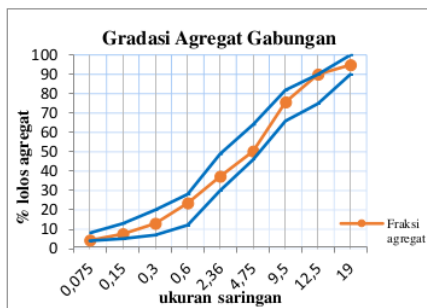
Gambar 10. Grafik fraksi agregat
