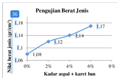
Gambar 7. Hasil uji berat jenis aspal
