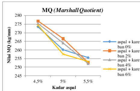
Gambar 16. Grafik nilai MQ
