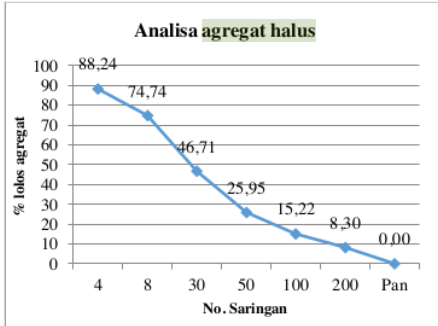
Gambar 8. Hasil analisa saringan agregat halus
