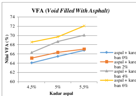
Gambar 13. Grafik nilai VFA
