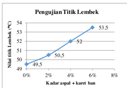
Gambar 3. Hasil pengujian titik lembek
