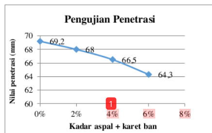
Gambar 2. Hasil penetrasi rata-rata
