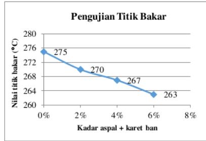
Gambar 6. Hasil pengujian titik bakar
