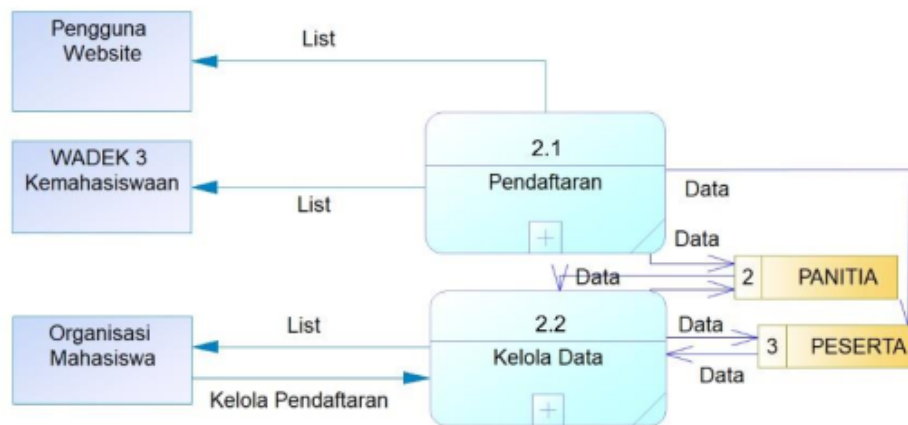
Gambar 3.5 DFD Level 2 Pendaftaran
