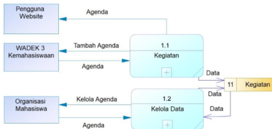
16 Gambar 3.4 DFD Level 2 Kegiatan
