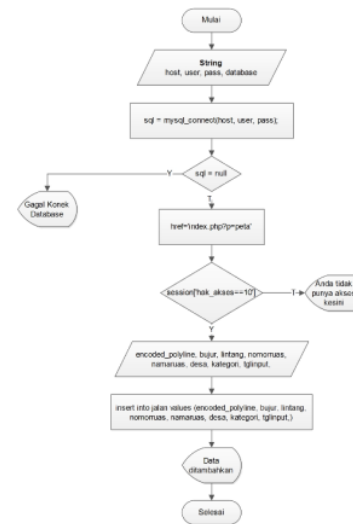
Gambar 13. Flowchart Pemetaan Jalan
