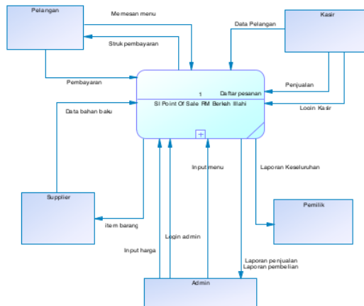
Gambar 5. Diagram Konteks
