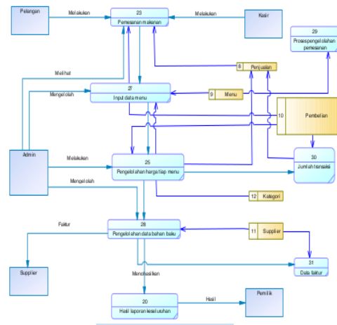
Gambar 7. DFD Level 2
