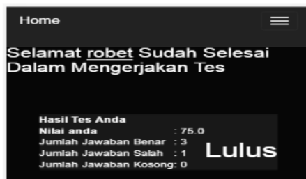
Gambar 18. Tampilan hasil
