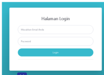
Gambar 3.4 Halaman Login
