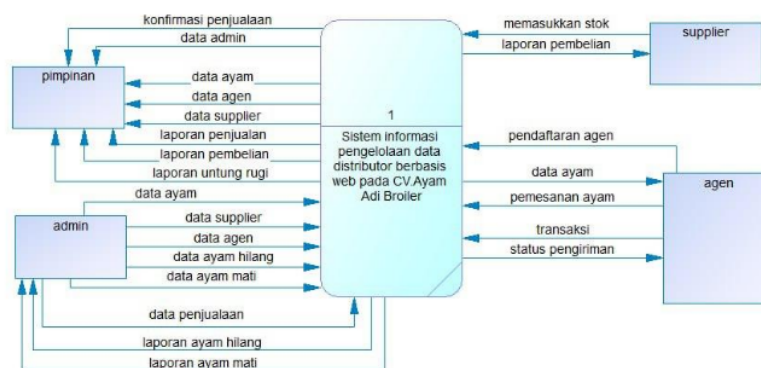
Gambar 3.1 Diagram Konteks
