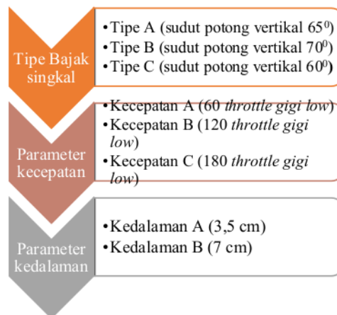
Gambar 3. 2 Parameter pengujian dengan soil bin
