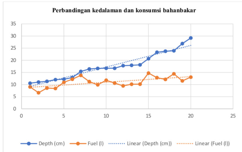
Gambar 4. 10 Grafik perbandingan Ketika ke dalam semakin dalam maka kebutuhan bahan bakar juga meningkat.
