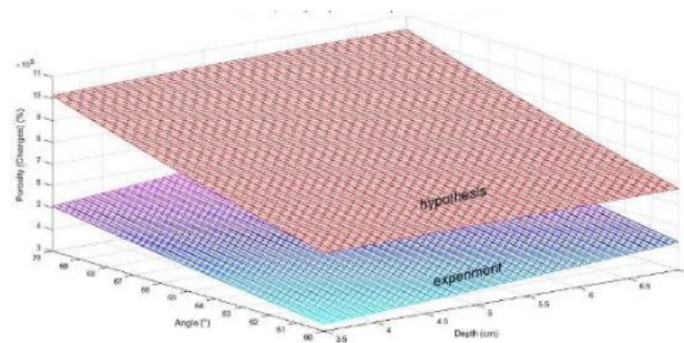
Gambar 2. 6 Grafik hasil percobaan berdasarkan pemodelan porositas tanah yang dipengaruhi oleh kecepatan pembajakan, sudut potong vertikal dan kedalaman pembajakan (Adisusilo, Hariadi, Yuniarno, et al., 2018).
