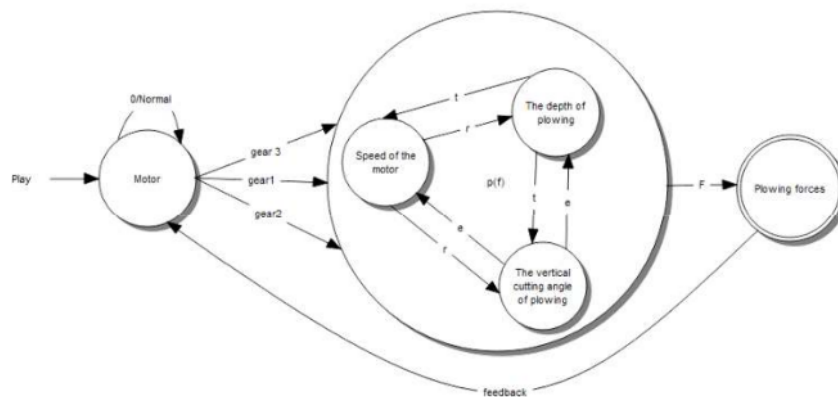
Gambar 2. 7 HFSM pengaruh kecepatan motor, sudut potong mata bajak dan kedalaman terhadap gaya tarik bajak singkal (Adisusilo, Hariadi, Mulyanto, et al., 2018).
