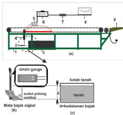
Gambar 3.8 (a).peralatan soil bin , (b). Letak strain gauge , (c). Tanah pada kotak dan kedalaman bajak sigkal.
