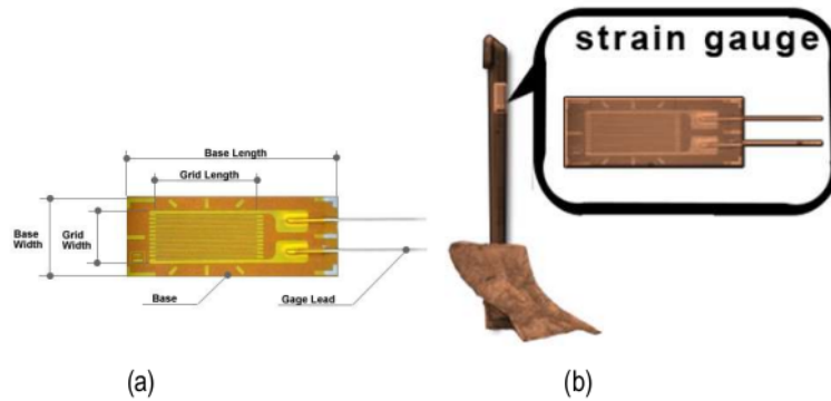
Gambar 3.5 (a). Strain gauge , (b) Posisi pemasangan strain gauge pada batang besi bajak singkal dalam percobaan soil bin .
