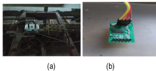
Gambar 3.7 (a).Jembatan wheatstone , (b). Strain amplifier dalam percobaan soil bin .
