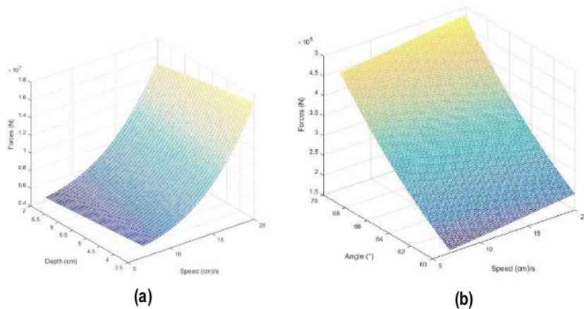
Gambar 2. 5 (a). Grafik hubungan kedalaman mata bajak dan kecepatan motor bajak terhadap gaya horizontal pada ordo ke-4. (b). Grafik hubungan sudut potong mata bajak dan kecepatan motor bajak terhadap gaya horizontal pada ordo ke-4 (Adisusilo, Hariadi, Mulyanto, et al., 2018).
