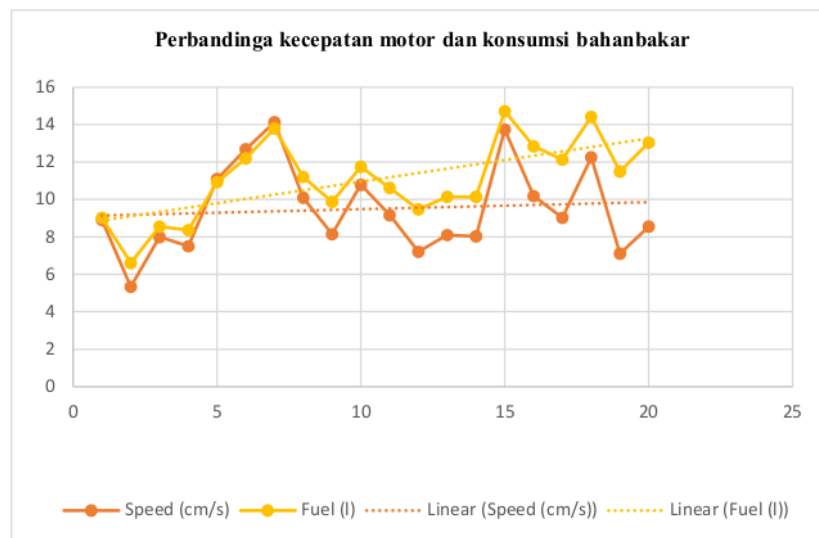
Gambar 4. 11 Grafik perbandingan kecepatan motor meningkat maka kebutuhan bahan bakar juga meningkat.
