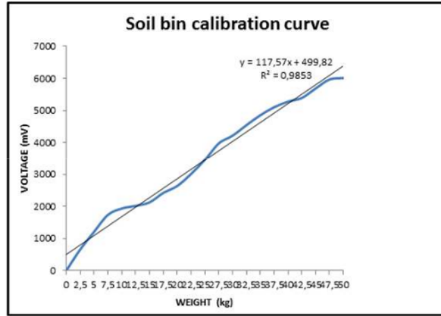
Gambar 2. 4 Kalibrasi untuk percobaan menggunakan soil bin
