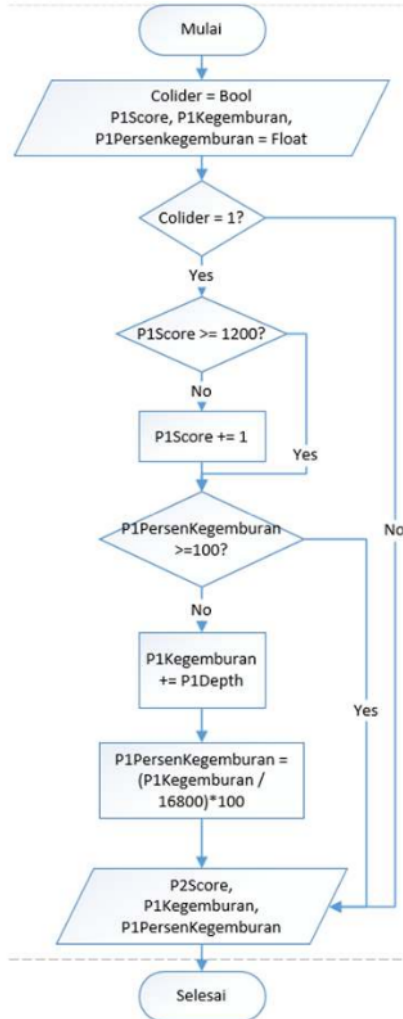
Gambar 4. 30 Flowchart p1score dan kegemburan
