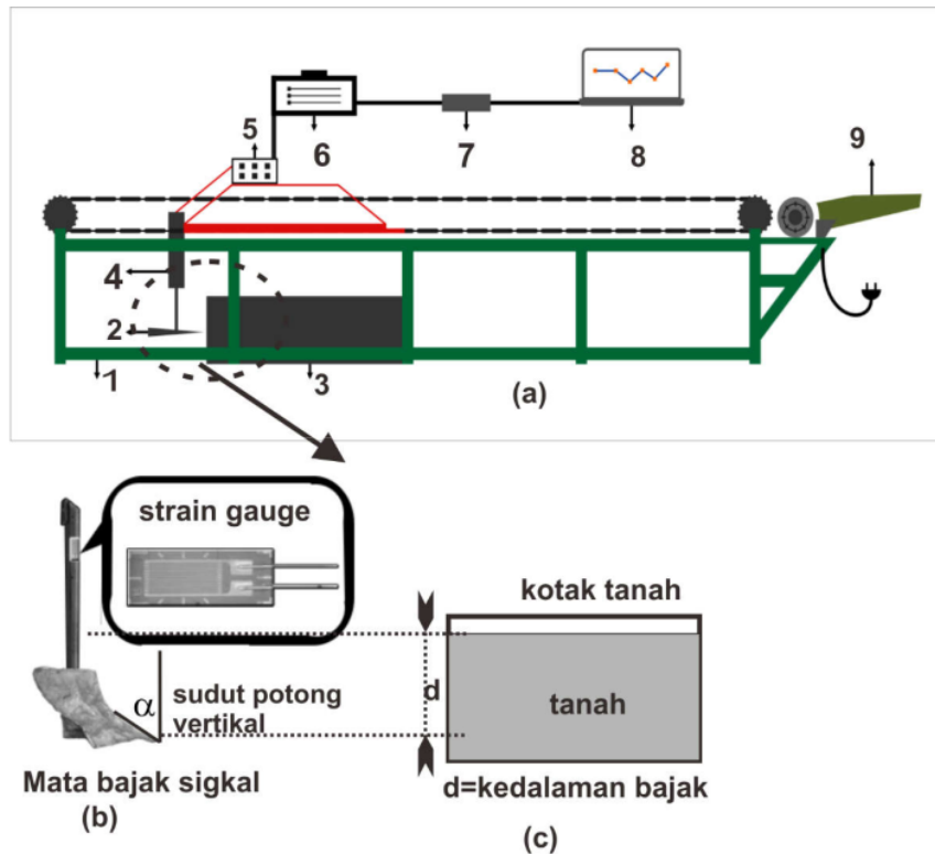
Gambar.3.8 (a).peralatan soil bin , (b). Letak strain gauge , (c). Tanah pada kotak dan kedalaman bajak sigkal.
