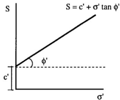
Gambar. 2.4. Grafik kekuatan geser tanah.
