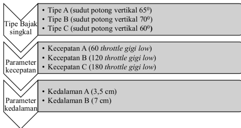
Gambar.3.2 Parameter pengujian dengan soil bin
