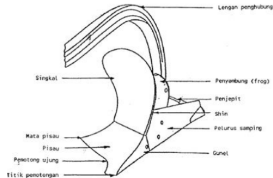
Gambar 2.6. Bagian bajak singkal satu bottom .
