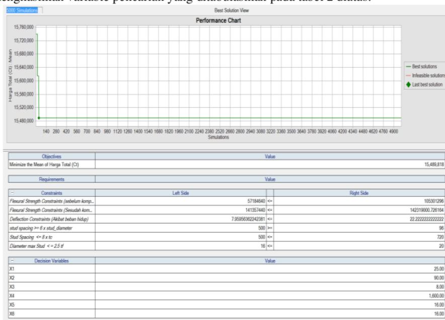
Gambar 7. Hasil Pencarian Metaheuristik OptQuest Scatter Search 5000 iterasi
