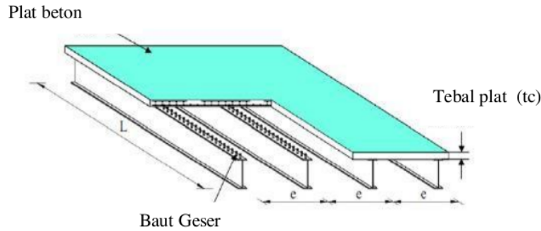
Gambar 4. Gambar Balok Komposit
