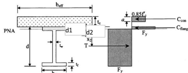
Gambar 5. Kapasitas Momen Komposit Balok ketika Plastik
