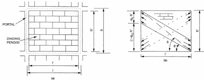
Gambar 3. (a) Portal Isi ; (b) Penopang Diagonal Bolak-balik
