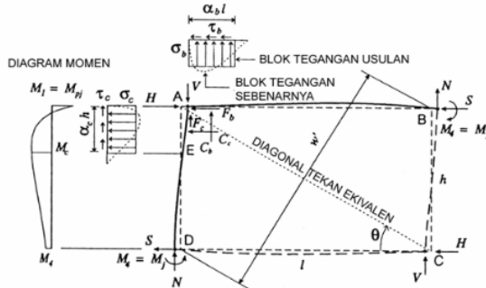
Gambar 5. Keseimbangan Gaya Pada Portal-Isi
