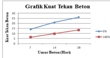
Gambar 4. Hasil Uji Kuat Tekan Beton
