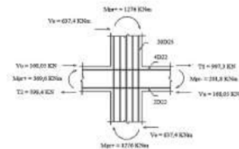
Gambar 8. HBK Terkekang 4 Balok
