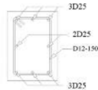
Gambar 15. Detail Penulangan Sloof
