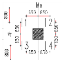
Gambar 13. Denah Kelompok Tiang Pancang Dinding Geser
