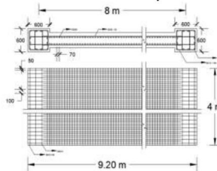
Gambar 11. Tulangan pada Dinding Geser dan Elemen Pembatas
