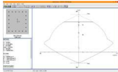
Gambar 5. Diagram Interaksi Kuat Rencana Kolom
