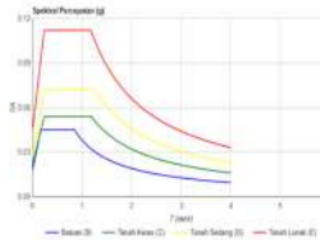
Gambar 3. Respon Spektrum
