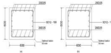
Gambar 7. Detail Penulangan Kolom
