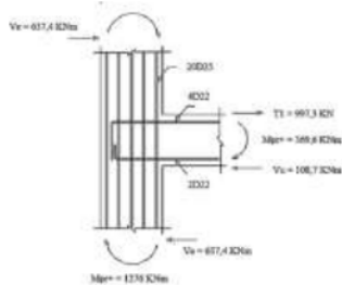
Gambar 9. HBK Terkekang 3 atau 2 Balok
