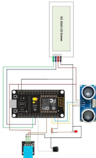
Gambar 4 rangkaian keseluruhan
