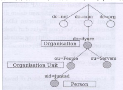
Gambar 1. Pohon Hirarki Direktori LDAP
